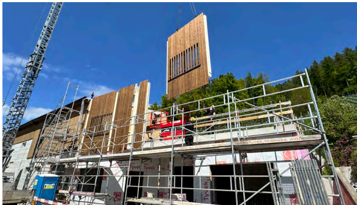
Eines der letzten Holzelemente findet seinen Platz im neuen Anbau des Ökonomiegebäudes auf dem Weingut Burkhart.
